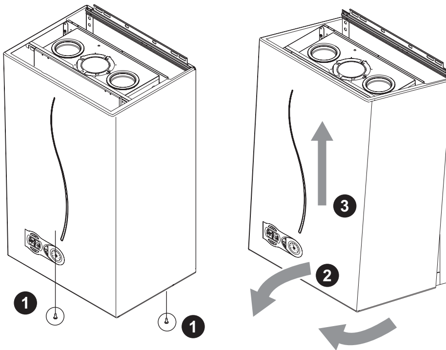
рис. 29 - Демонтаж кожуха
