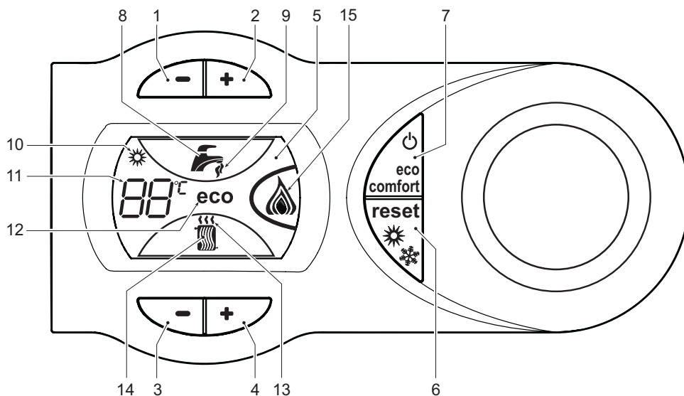
рис. 1 - Панель управления
