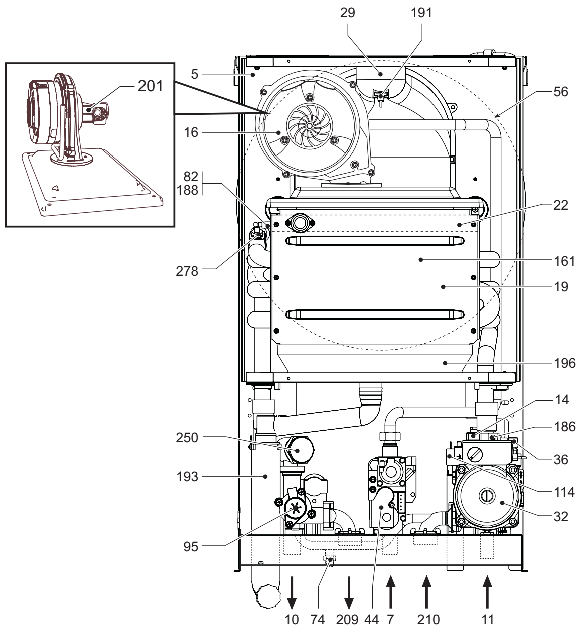
рис. 32 - Общий вид
