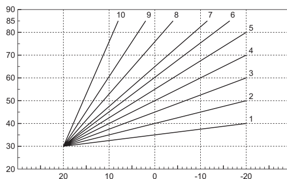
рис. 12 - Компенсационные характеристики
