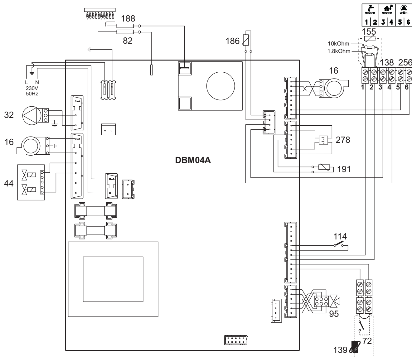
рис. 34 - Электрическая схема
