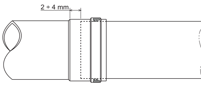
рис. 20 - Тепловое расширение
